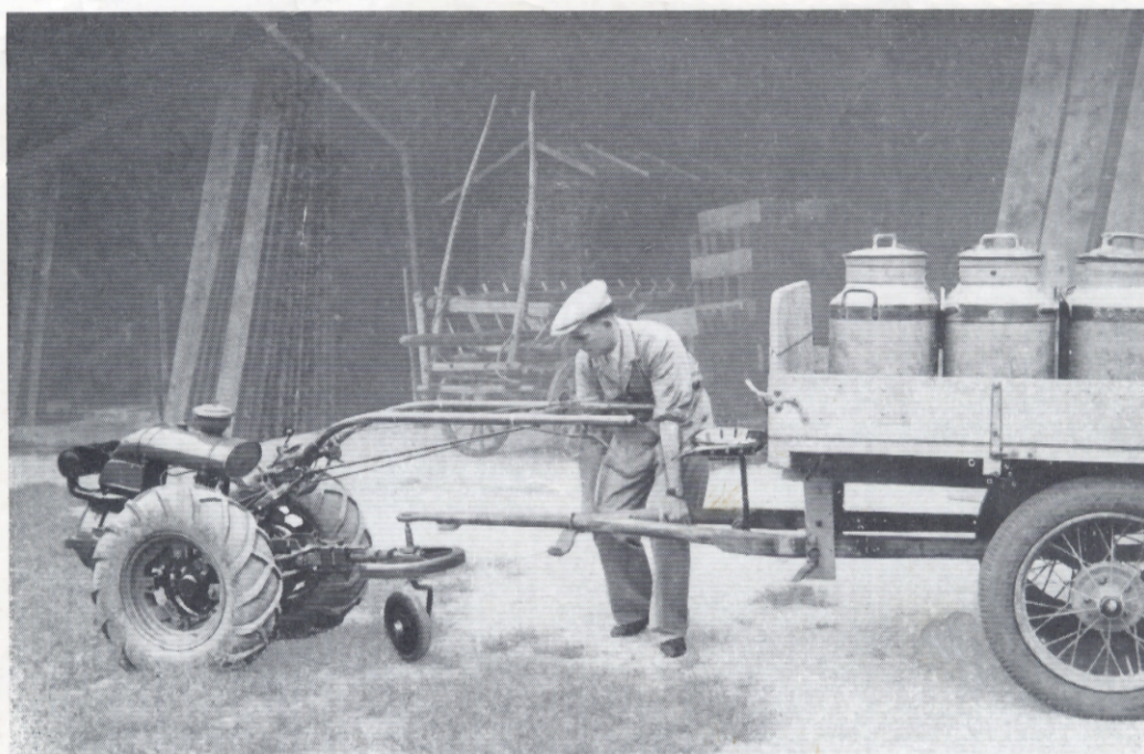
Motoculteur 60 A Accouplement d'une remorque sur bras de traction élastique. Landwirtschaftsmaschine 60 A Ankupplung eines Anhängers auf elastischem Zugarm.
