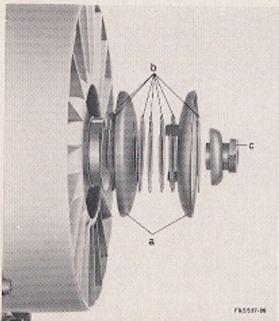
Figure 13: a) flasque de la poulie b) rondelles d'épaisseur c) écrou de blocage
