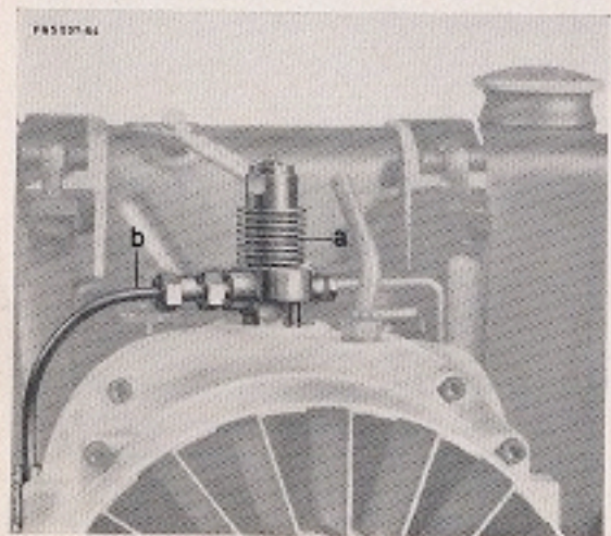
Figure 19: a) injecteur positionné pour essai b) conduite haute pression
