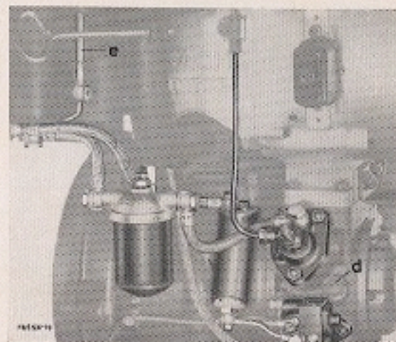
Figure 11: d) bouchon de remplissage d'huile du porte-accessoires e) niveau d'huile sur le réservoir
