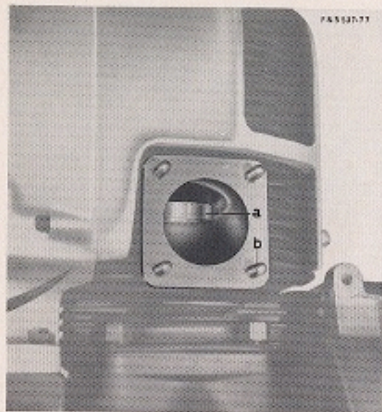
Figure 18: a) piston se trouvant 10 mm au dessus du point mort bas b) fixation du pot d'échappement
