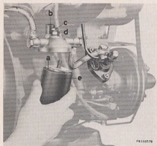
Figure 16: a) cartouche de filtre b) vis de purge de la partie extérieure du filtre c) vis de purge de la partie intérieure du filtre d) vis creuse de fixation de la cuve de filtre e) cuve de filtre
