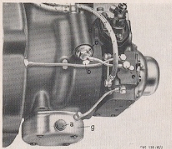
Figure 15: a) bouchon de vidange d'huile b) vis creuse c) écrou à pans du filtre à huile d) tuyau de retour d'huile de la pompe au réservoir e) vis creuse f) tuyau d'huile du filtre à la pompe g) réservoir de récupération d'huile
