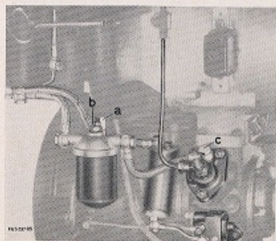
Figure 20: a) vis de purge de la partie extérieure du filtre b) vis de purge de la partie intérieure du filtre c) vis creuse sur la pompe d'injection
