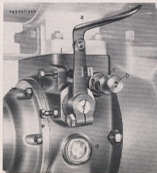
Figure 3: Points de réglage et de commande du moteur a) Levier d'accélération b) bouton de démarrage c) limiteur de fumée d) niveau d'huile e) vis de réglage du nombre maximum de tours f) vis de réglage du ralenti i) ressort à lames sur le levier d'accélération.
