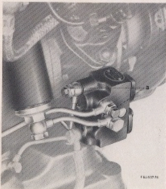
Figure 21: a) vis bouchon pour vis creuse
