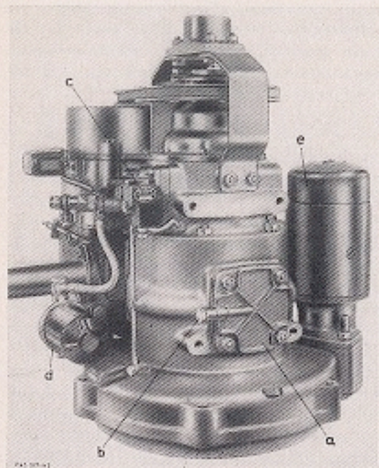
Figure 9: a) couvercle du carter de vilebrequin b) raccord pour tuyau de récupération d'huile c) pompe de huile d) filtre à combustible e) démarreur
