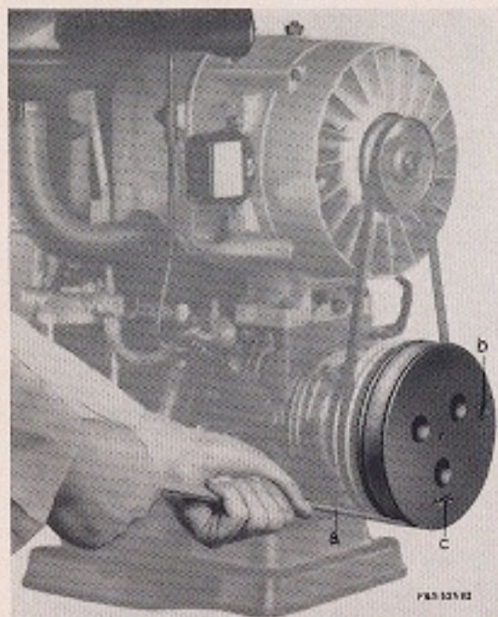
Figure 6: Démarrage avec poulie et courroie a) Courroie b) Emplacement de la poignée c) Sens de rotation
