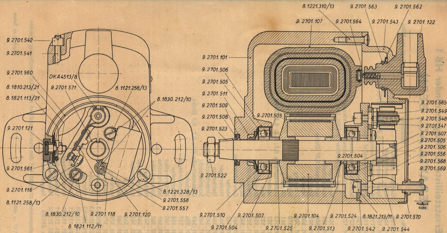
Schnitt
