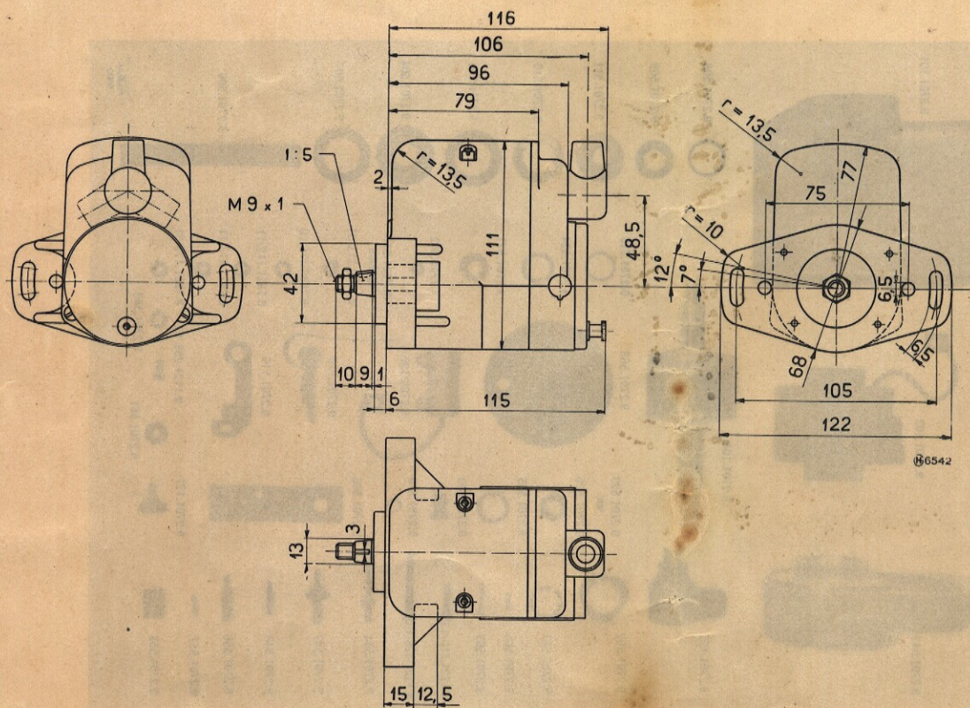
Masszeichnung
